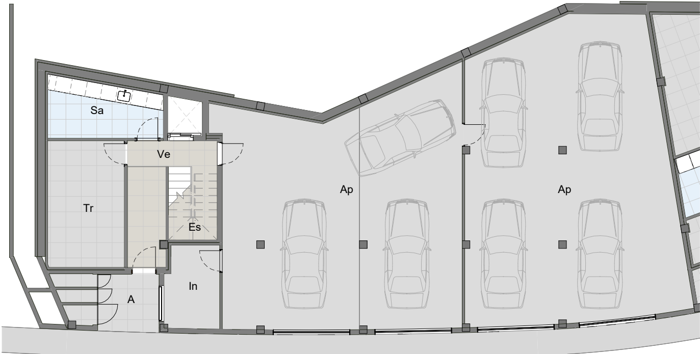
1 Xalet 2 - P-1 - Venda 1 : 150
